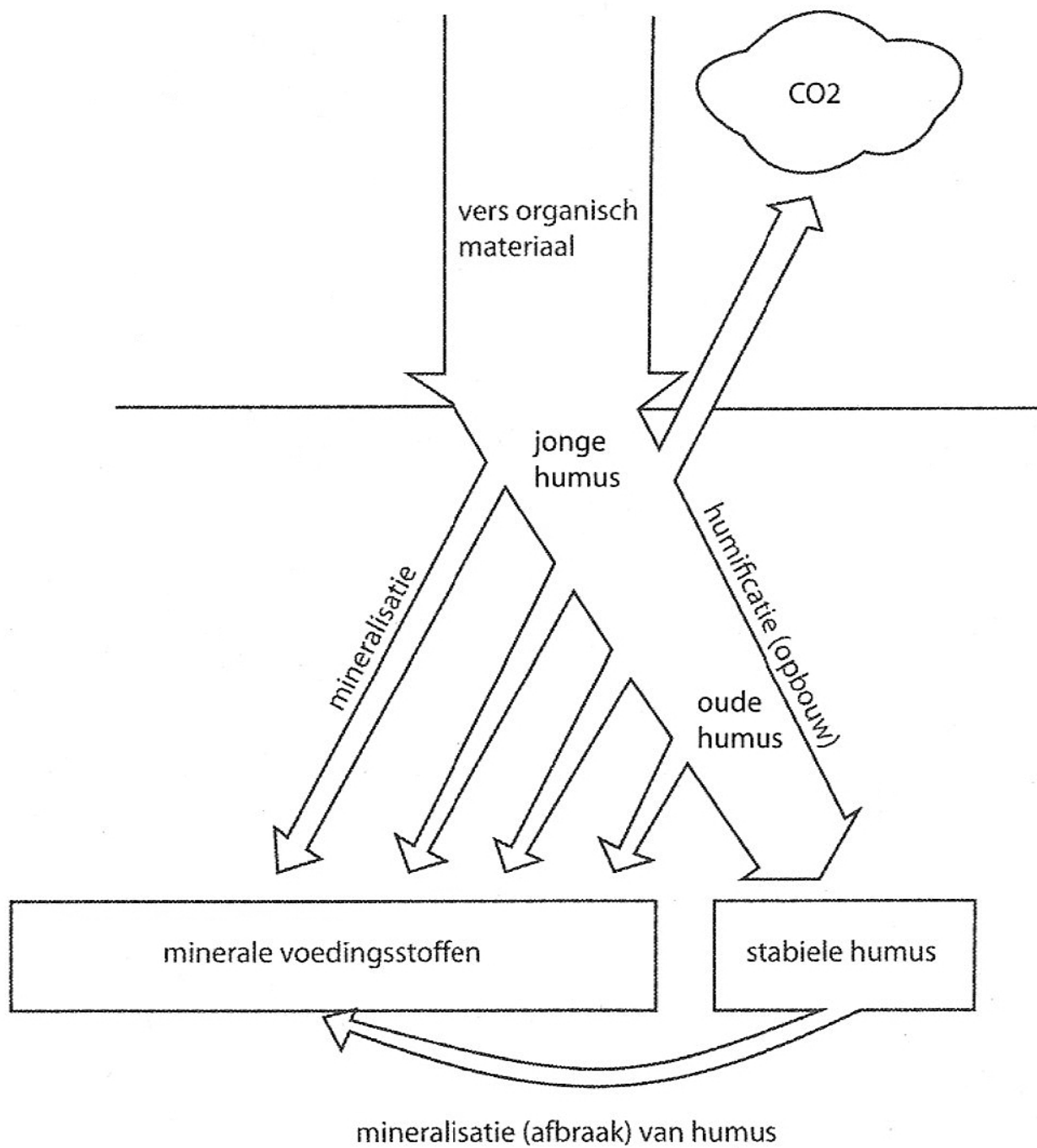
Tekening 4.6. Mineralisatie en humificatie
